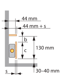
Plintverwarming Mini Classic
