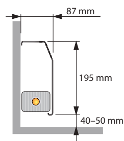
Plintverwarming IIa Delta
