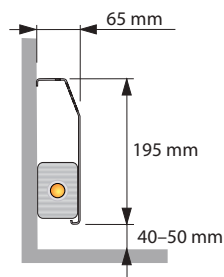
Plintverwarming Ia Delta
