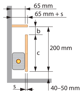
Plintverwarming Ia Classic
