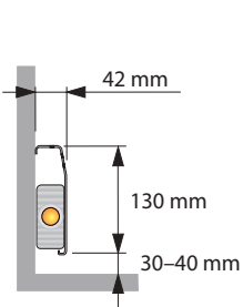
Plintverwarming Mini Delta
